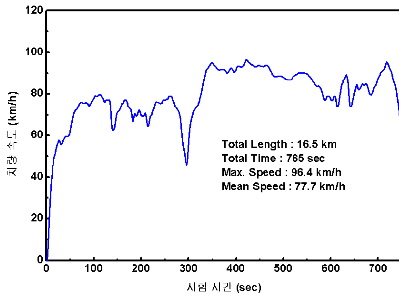
[그림 7] HWFET 주행시험 계획
